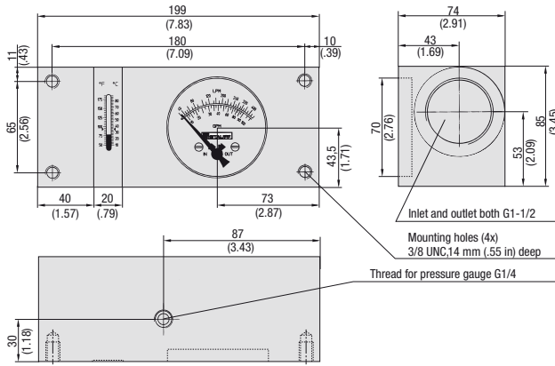
Dimensions SDM-1500
