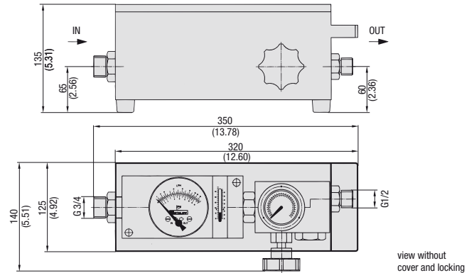
Dimensions SDM-K-750
